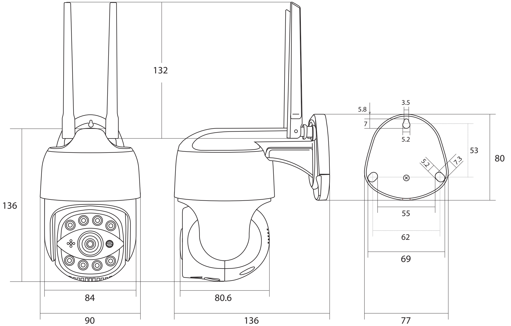
図名 500万画素 IP 防犯灯パンチルトカメラ 図番 WTW-E2305GX/GBX WIRELESS TSUKAMOTO CO., LTD
