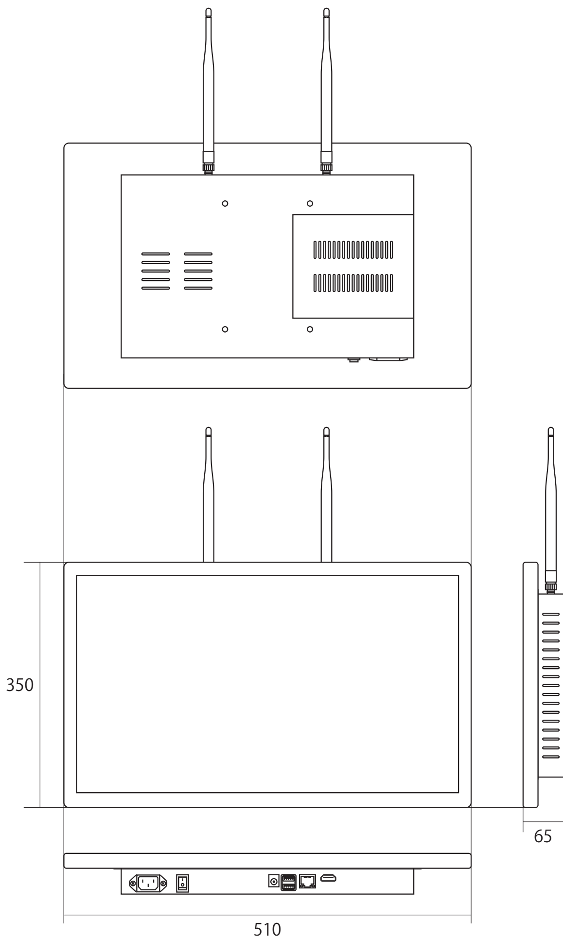
図名 IPカメラシリーズ用 10CHデジタルレコーダー 図番 WTW-EG2610WHAX-22 WIRELESS TSUKAMOTO CO., LTD
