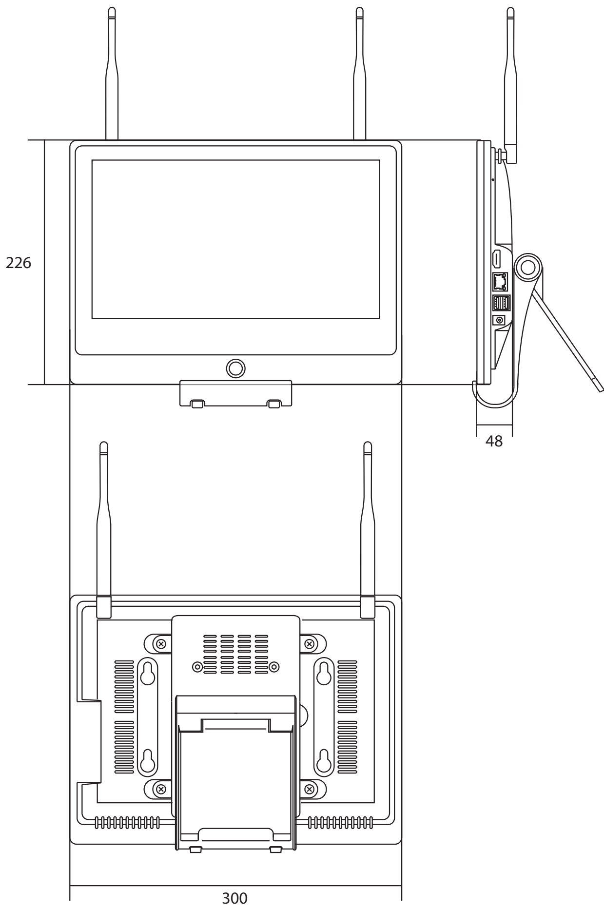
図名 WiFi IPカメラ用 16CHデジタルレコーダー 図番 WTW-EG2616WHAX WIRELESS TSUKAMOTO CO., LTD
