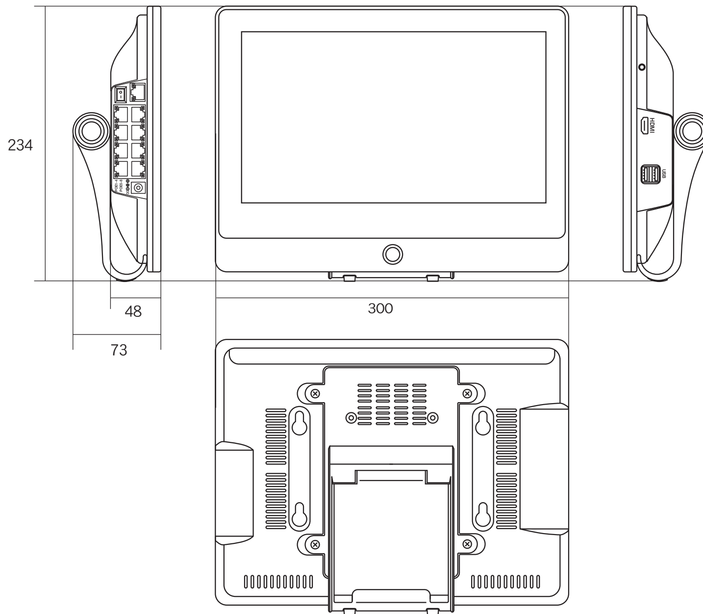
図名 XPoE 16ch対応 12インチモニター内蔵 (NVR) 図番 WTW-BNV270EPL/GPL
